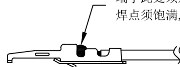
端子点锡示意图 △
